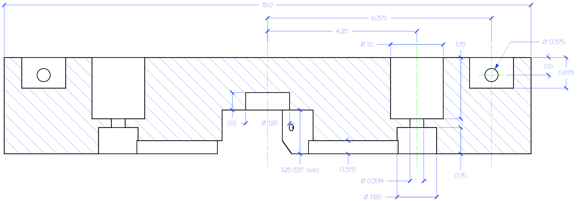
Section A-A -scale 3:4
