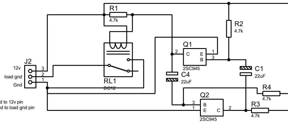
12v Universal Flasher
